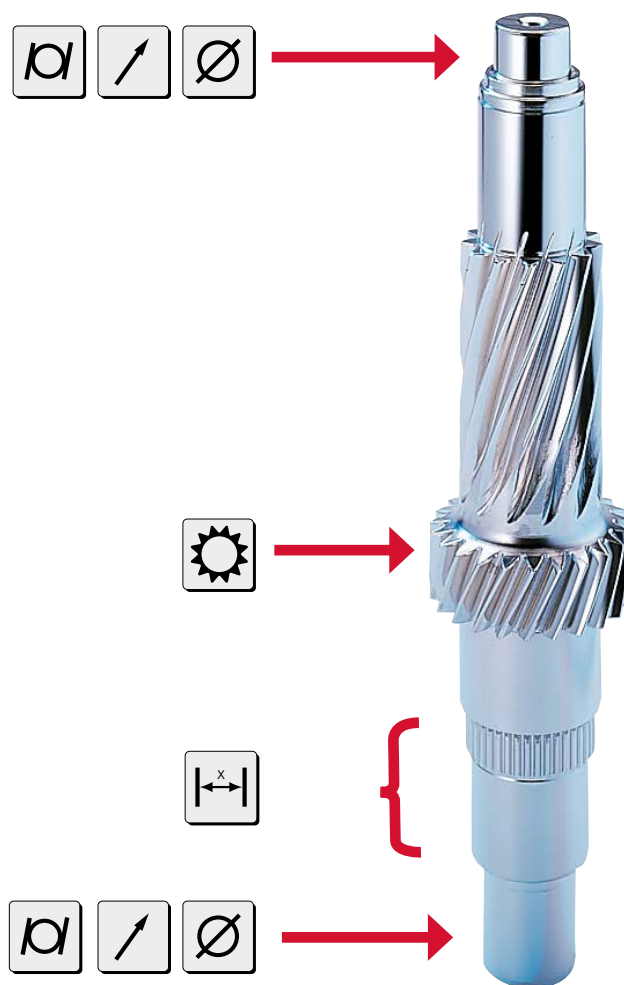
Beispielhafte Messaufgaben an einer Schaltgetriebewelle
